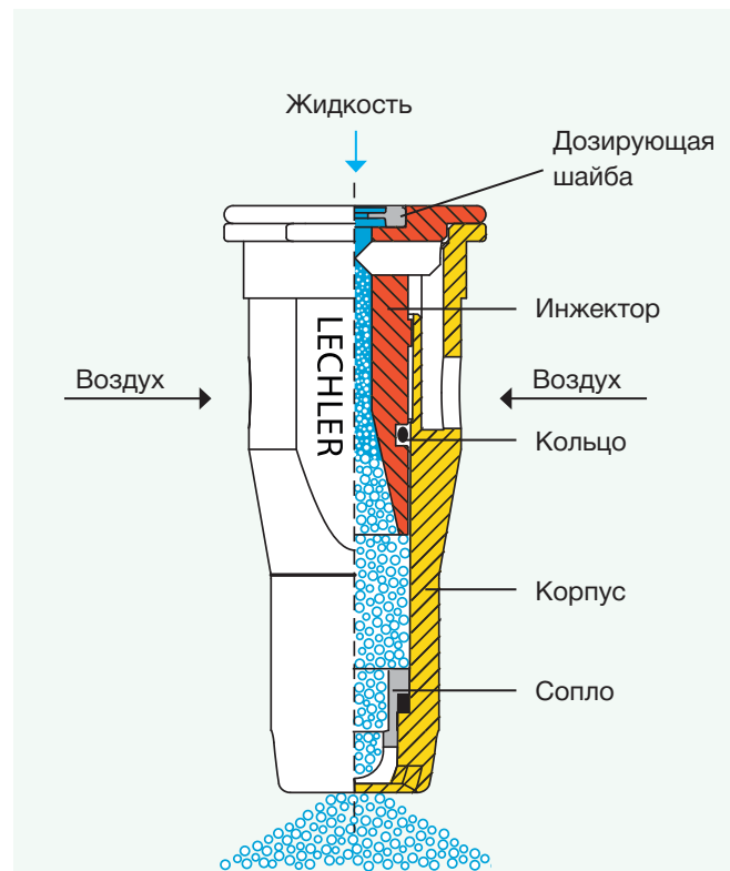
Схема работы форсунки ID3
